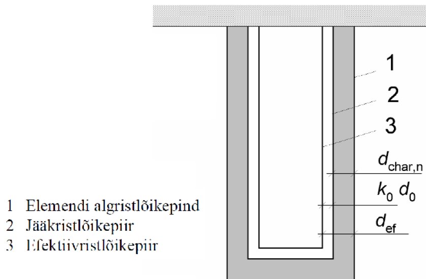
Joonis 6. Jääkristlõike ja efektiivristlõike määratlus. (Eesti Standardikeskus, 2007, p. 35)
