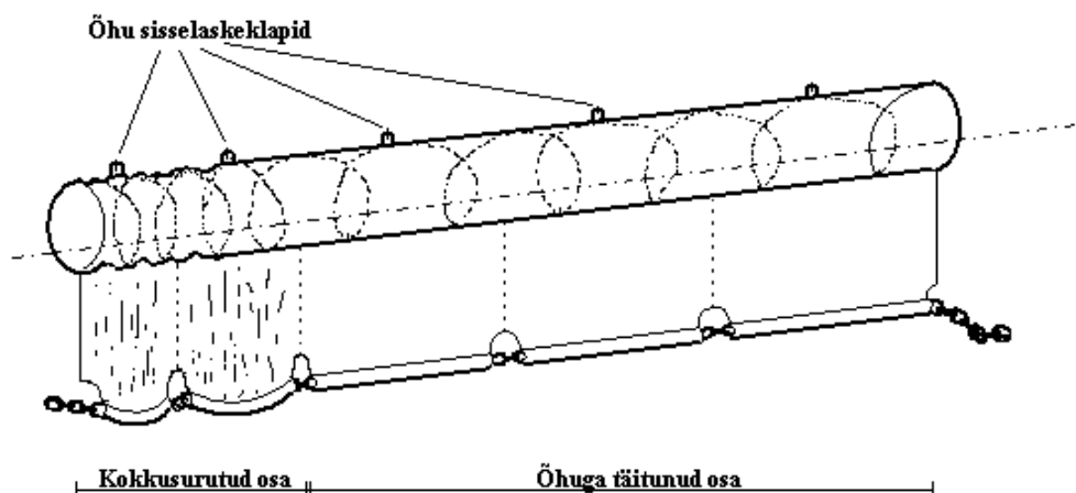
Joonis 4 - Isetäituv ujuvpoom.
