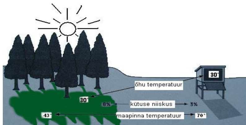
Joonis 14. Varju mõju pinnakütuste temperatuurile ja niiskusele (Lowe 2001:25)
