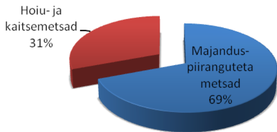
Joonis 6. Metsa pindalane kasutamine (Adermann 2006:21)
